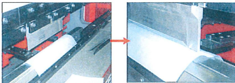
使用例1 (SUS430 鏡面材 1.2t P/D=88° V=10 mm)
