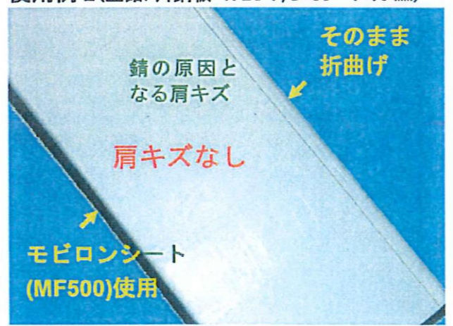
使用例2 (亜鉛メッキ鋼板 1.2t P/D=88° V=10 mm)
