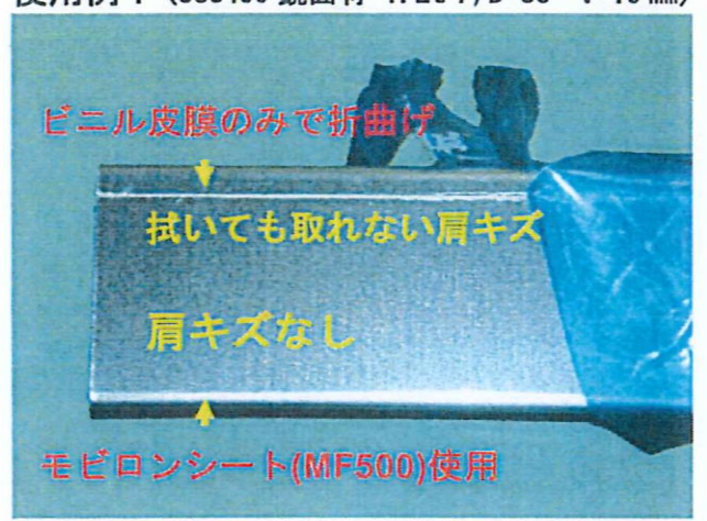
使用例1 (SUS430 鏡面材 1.2t P/D=88° V=10 mm)
